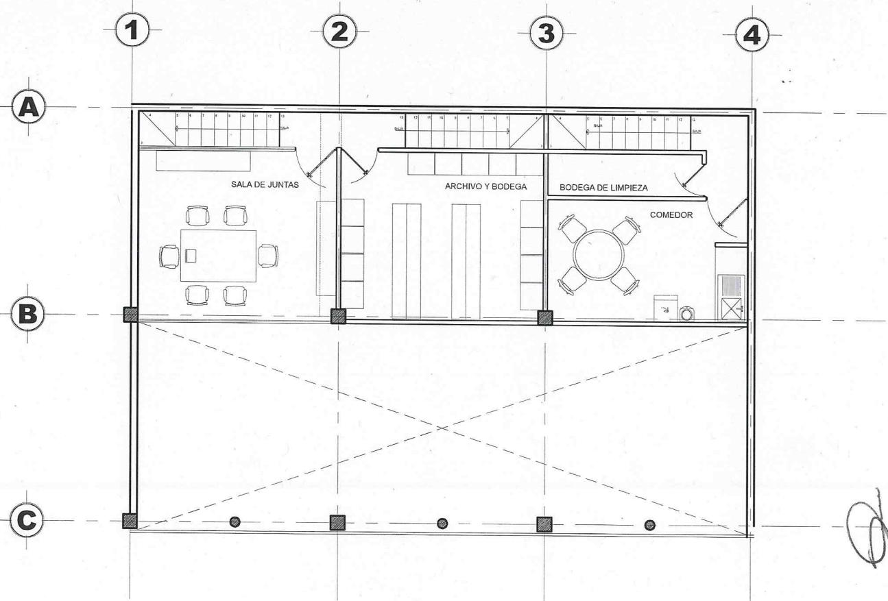
PLANTA ALTA
